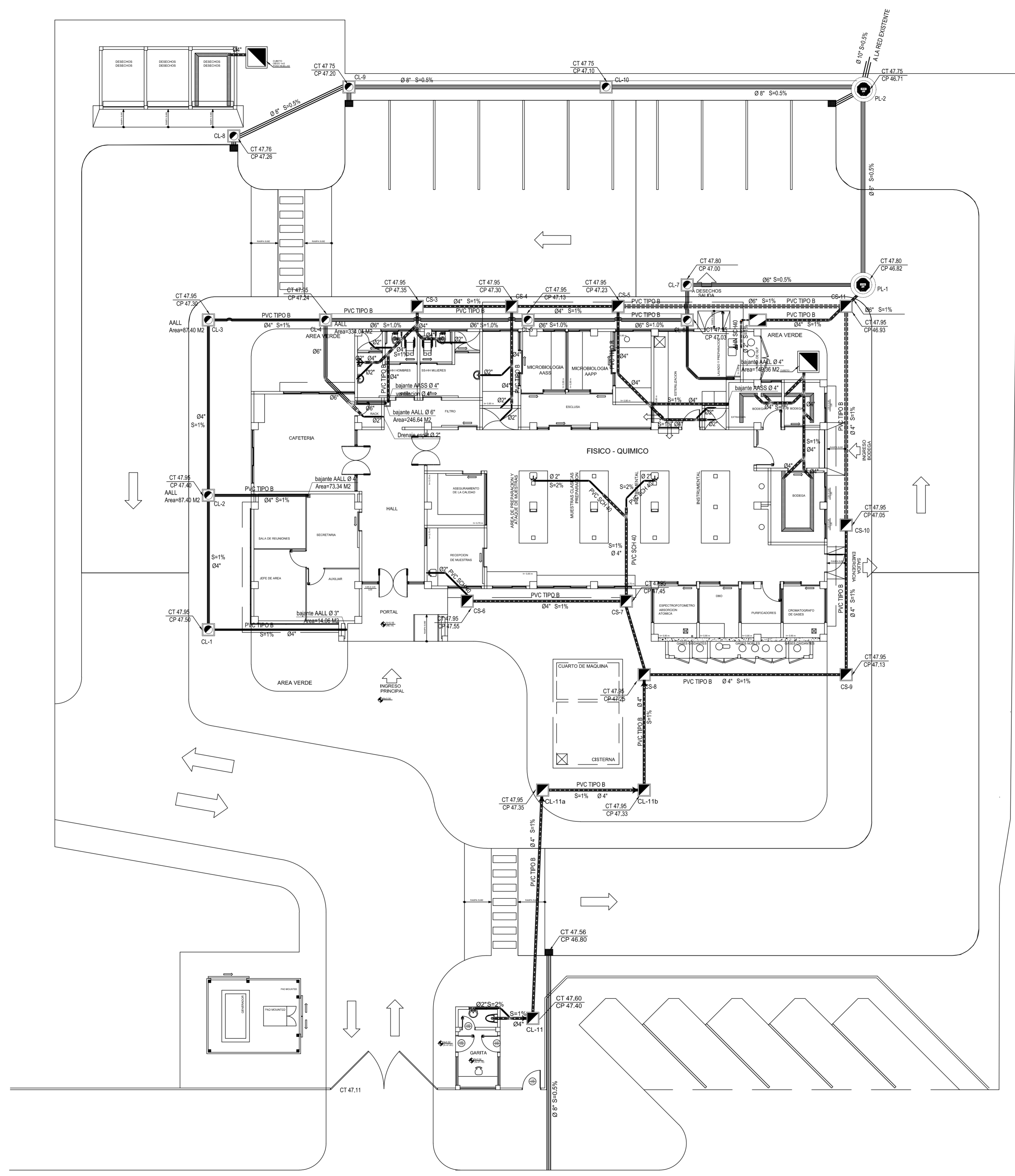
1 PLANTA SISTEMA AA.SS Y AA.LL. NIVEL +0.18 Scale: 1:125
